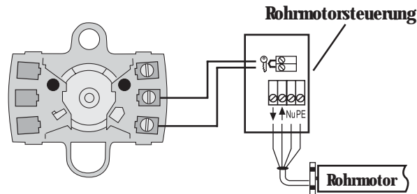
Anschlussbild für Rohrmotorsteuerung
