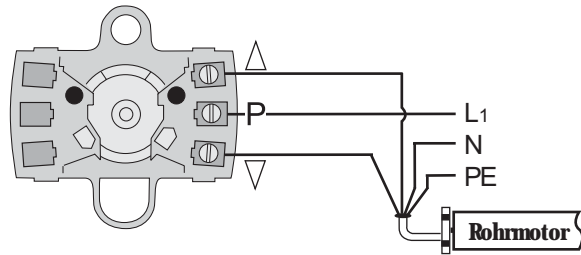
Anschlussbild für 1 Rohrmotor
